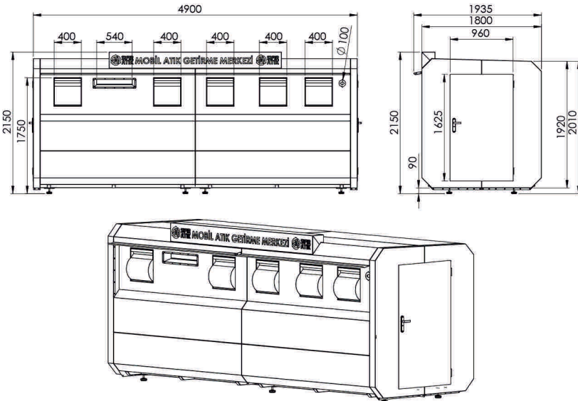
2.SINIF ATIK GETİRME MERKEZİ TEKNİK ÖLÇÜLERİ
