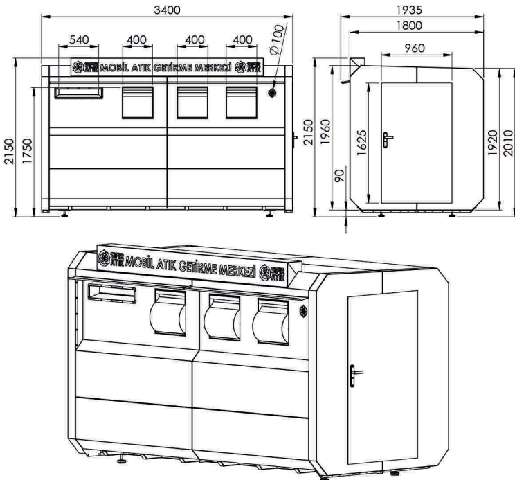
3.SINIF ATIK GETİRME MERKEZİ TEKNİK ÖLÇÜLERİ
