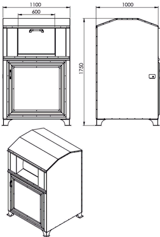
AMBALAJ ATIKLARI KUMBARASI TEKNİK ÖLÇÜLERİ
